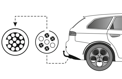
Thule Adapter 9906 – Adapter zwischen 7-poliger Steckdose des Fahrzeugs und 13-poligem Stecker.
