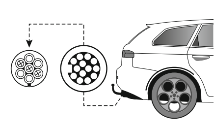
Thule Adapter 9907 – Adapter zwischen 13-poliger Steckdose des Fahrzeugs und 7-poligem Stecker.
